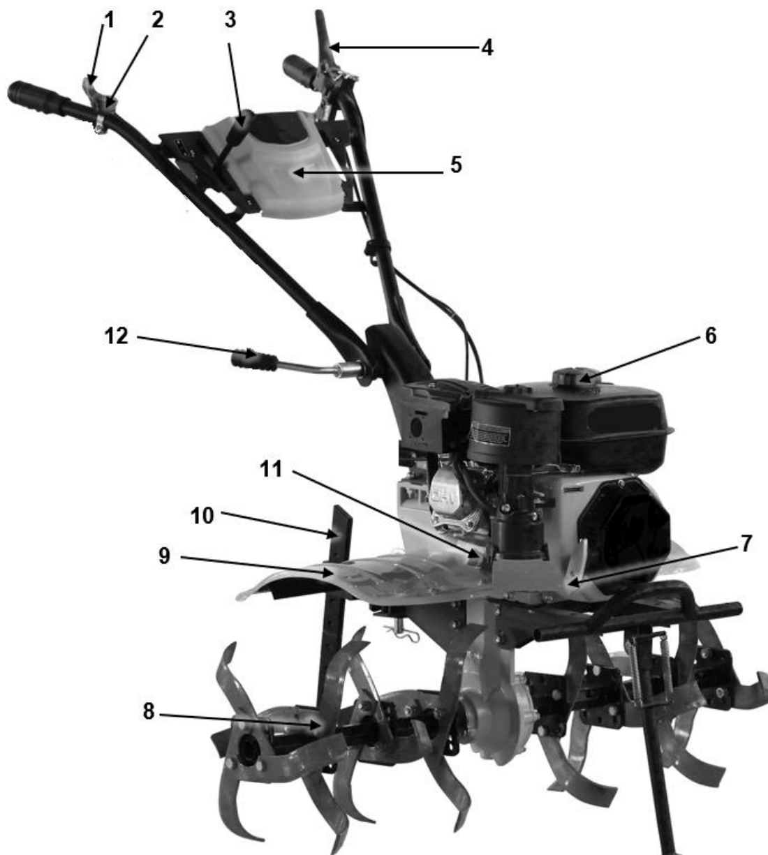
Рисунок 1 – Основные части и узлы культиватора
