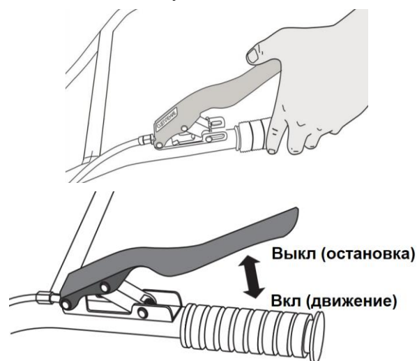
Рисунок 7 – Рычаг сцепления
