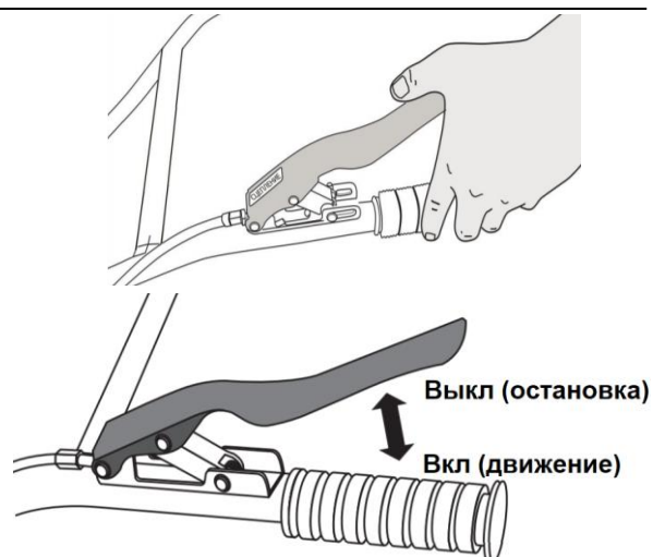
Рисунок 7 – Рычаг сцепления
