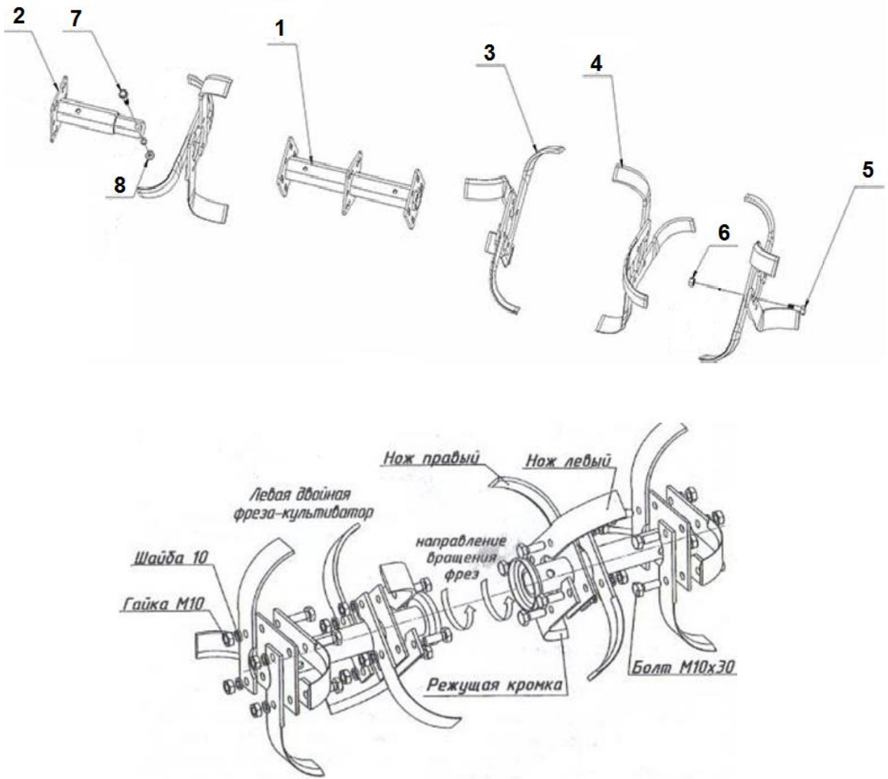
Рисунок 3 – Сборка фрез
