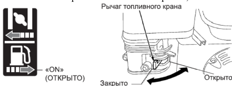
Рисунок 9 – Топливный кран
