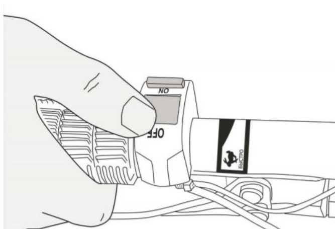
Рисунок 16– Выключатель двигателя
