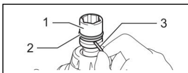
1-ударная головка 2-Уплотнительное кольцо 3-Штифт
