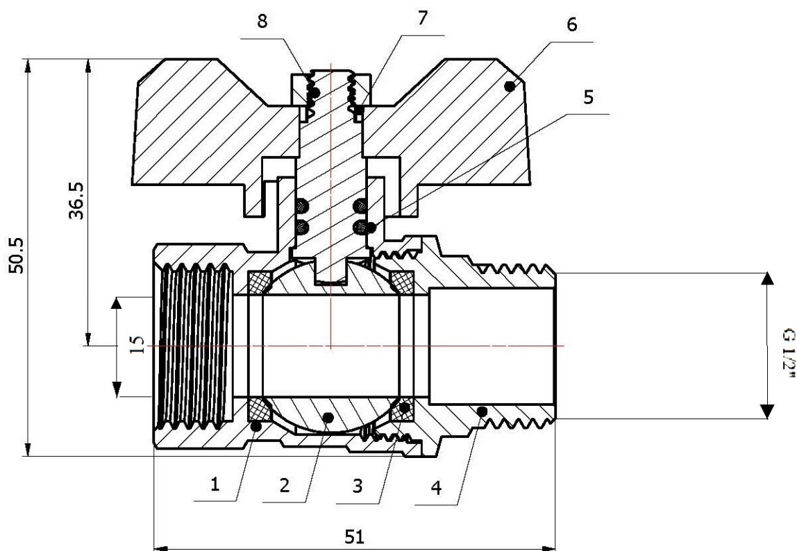
Рис.2. Габариты крана 1/2"
