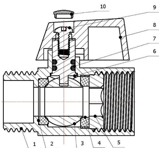
Рис.1. Общий вид шарового крана
