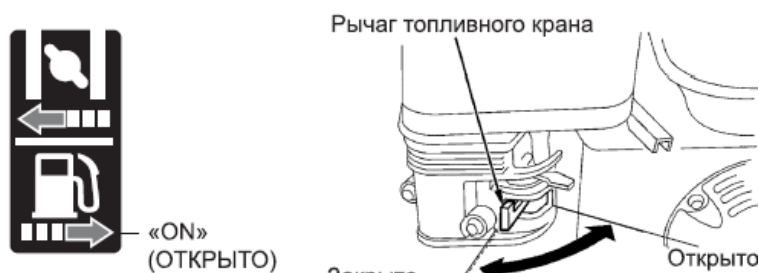
Рисунок 9 – Топливный кран
