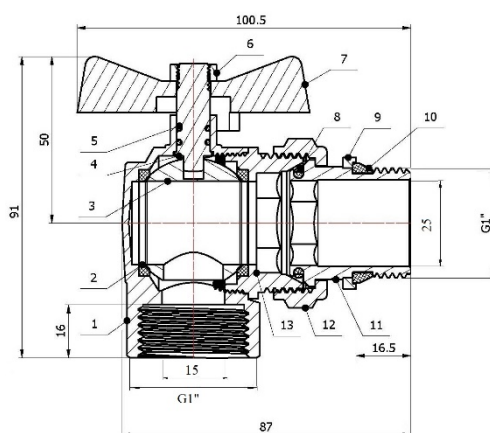
Рис.3. Габариты крана 3/4", арт. AVE094034E
