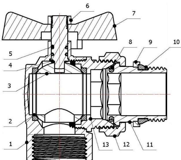
Рис.1. Общий вид шарового крана
