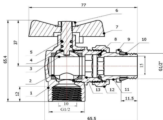
Рис.2. Габариты крана 1/2", арт. AVE094012E
