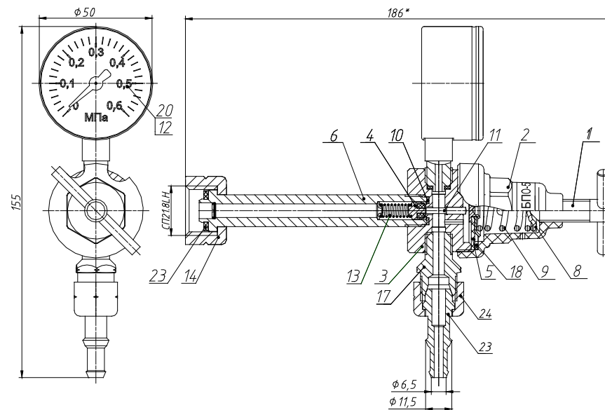
Рис. 1. Редуктор баллонный пропановый одноступенчатый (с удлиненным штуцером).
